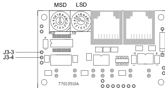
G2 LightSync Controller
