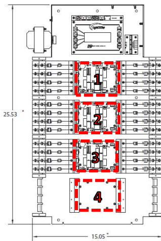
LLZMAXRI-24 Retrofit Insert (Enclosure 34" x 20" x 4")
