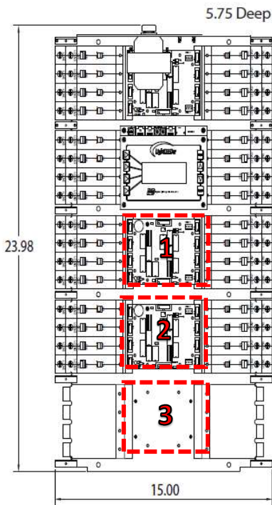
LightLEEDer-32 Retrofit Insert
