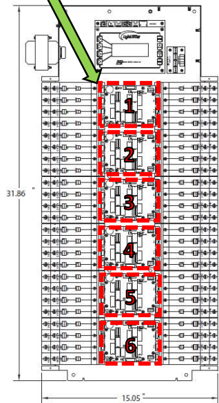
LLZMAXRI-48 Retrofit Insert (Enclosure 54" x 20" x 4")
